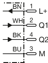
接线图
