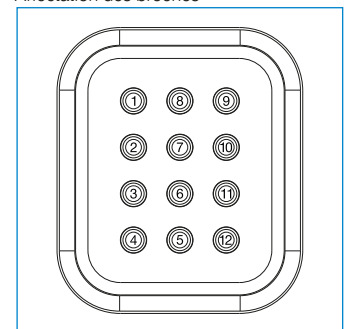
Affectation des broches
