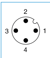
Obłożenie PIN-ów
