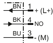
接线图
