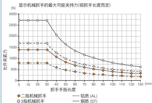
▶ 夹持力图表
