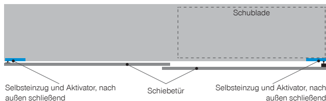
Schrank, geschlossen
