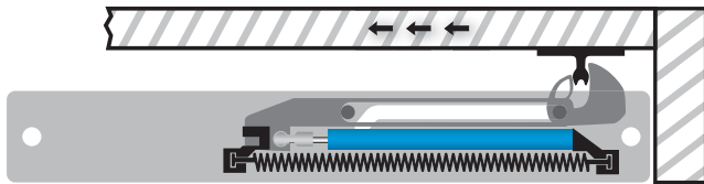
Tür geschlossen
