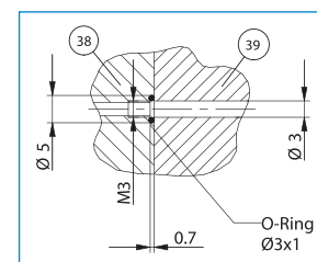
无软管空气传输(工具端)
