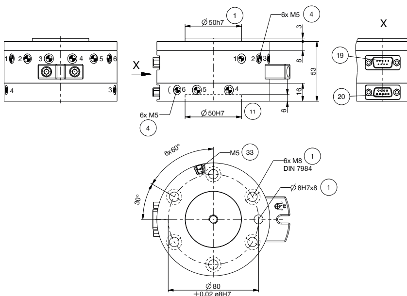
无软管空气传输(工具端)
