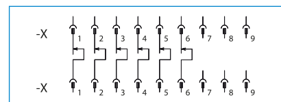
PIN分配
